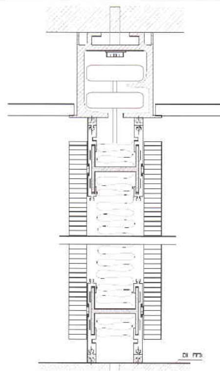
Řez systému
